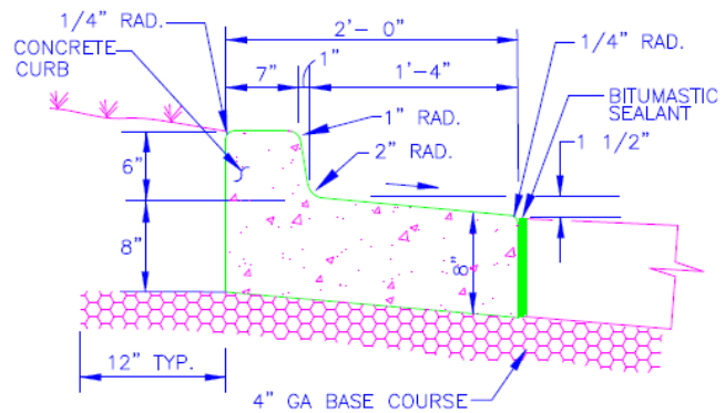
CURB/WITH SPILL GUTTER
